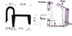
HB-335 顶部构件 Top panel retainer
