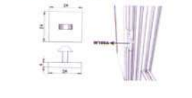
HB-337 中间用托件 Panel retainer for horizontal grooves
